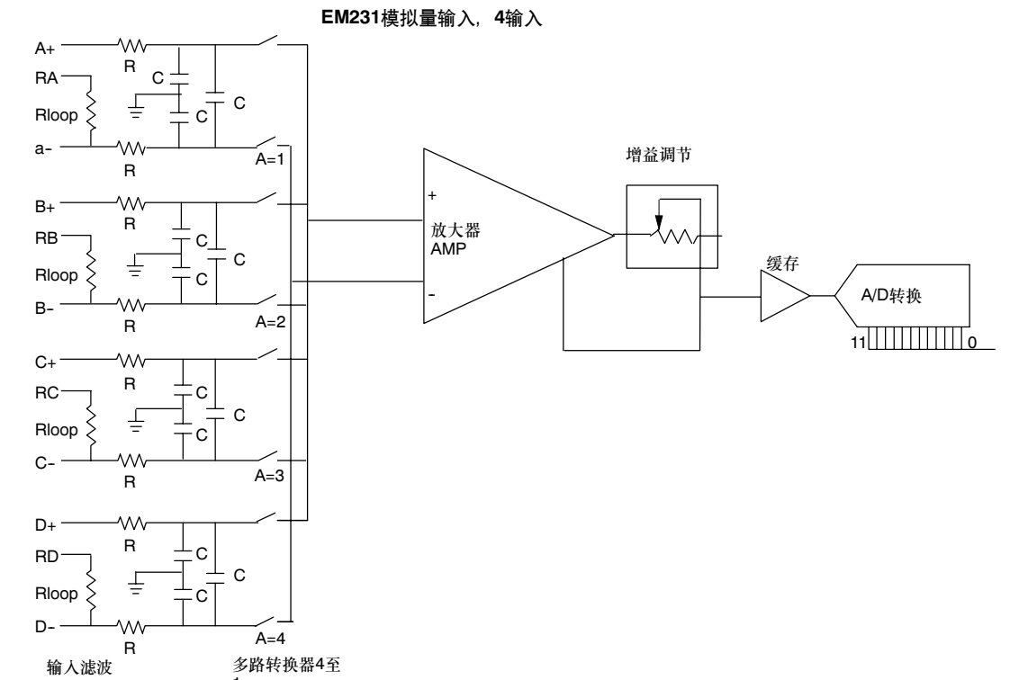
图A-17 EM 231 模拟量输入的输入方框图, 4输入
