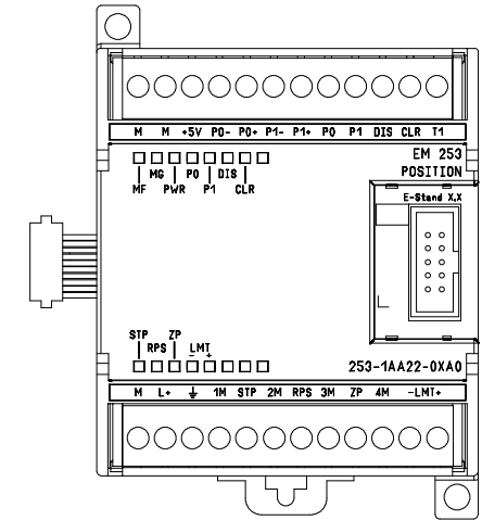
图9-9 EM253位控模块
