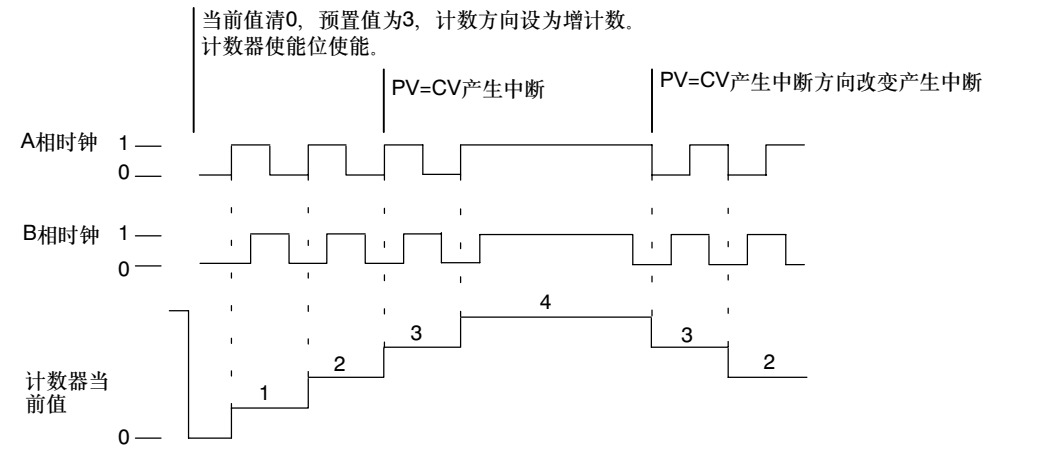
图6-25 模式9、10或者11操作实例（一倍速正交模式）
