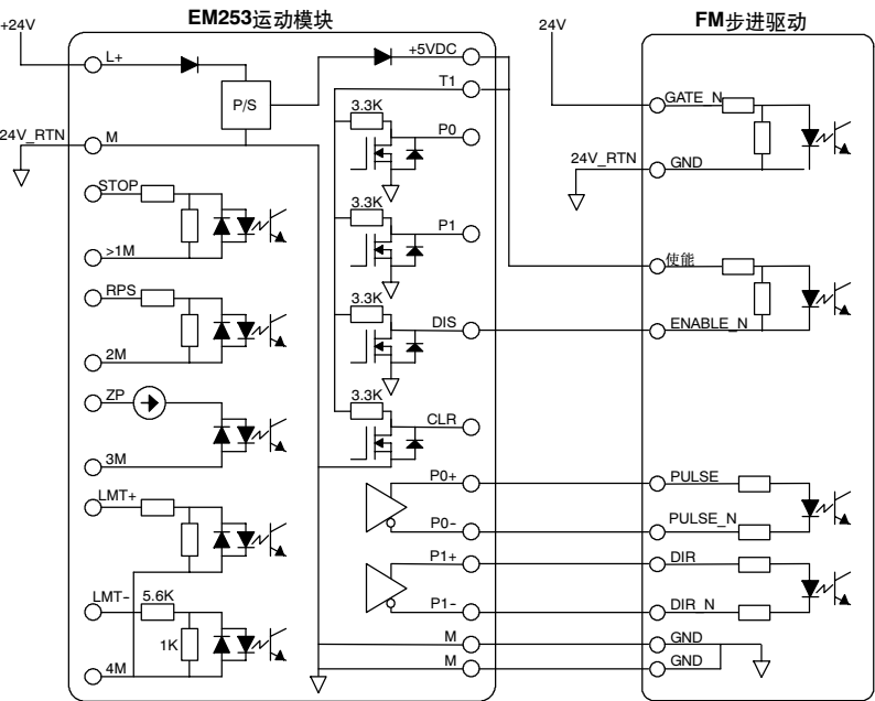
图A-36 连接EM253位控模块和FM步进驱动
