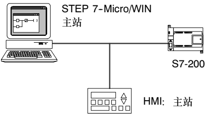
图7-7 PPI网络
