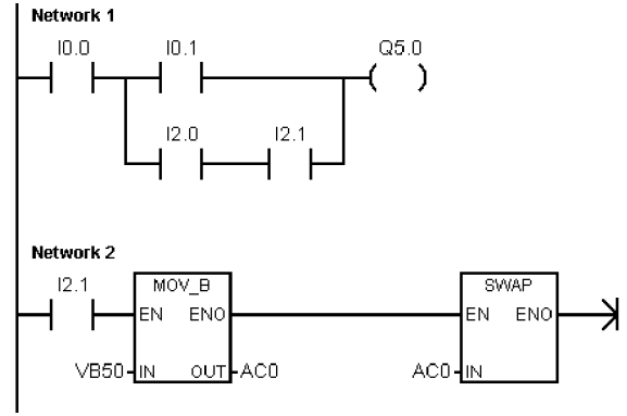
图5-3 LAD程序示例
