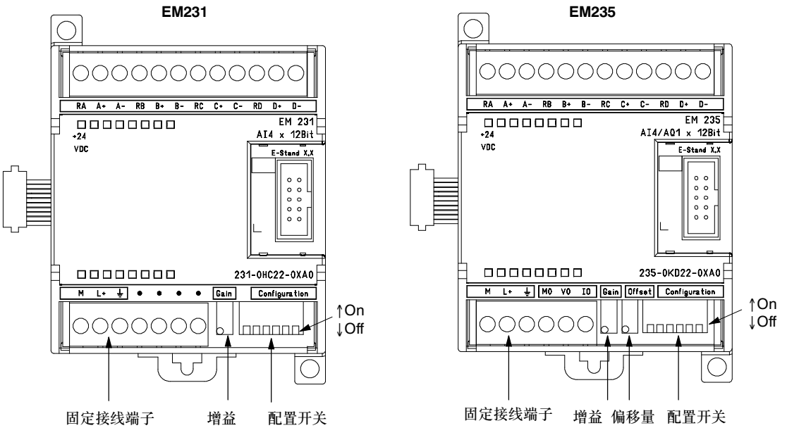
图A-15 EM231和EM235校准电位计和配置DIP开关位置
