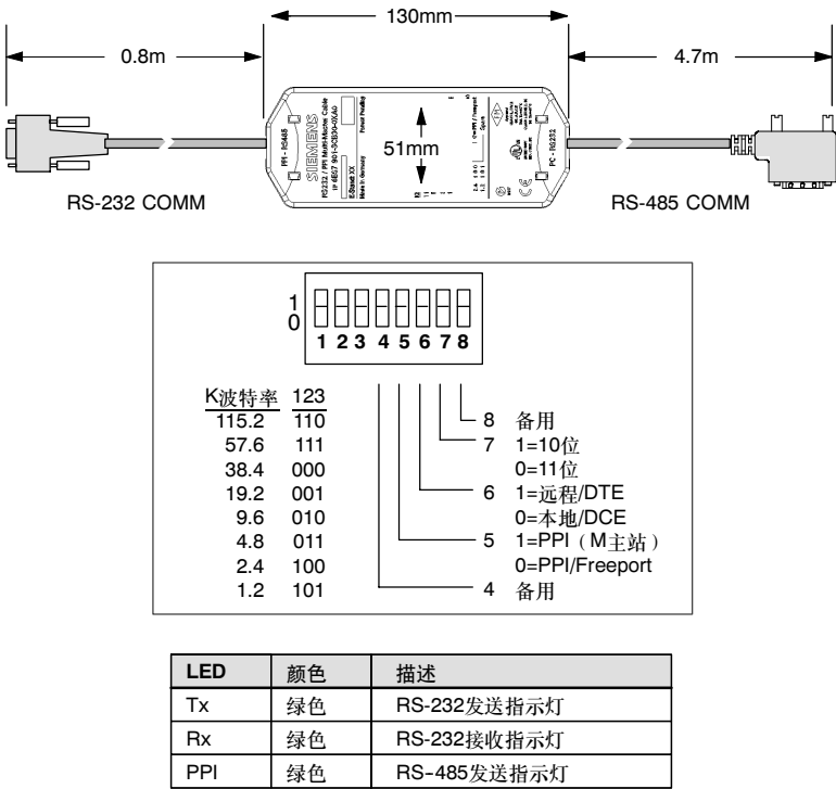
图A-44 S7-200 RS-232/PPI多主站电缆的尺寸、标签和LED
