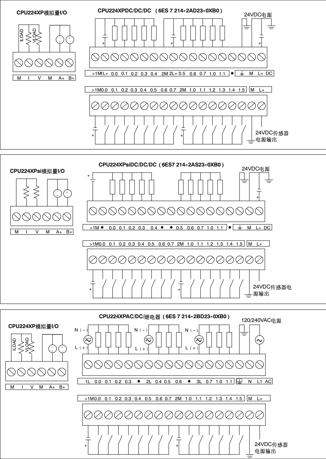
图A-5 CPU 224XP接线图
