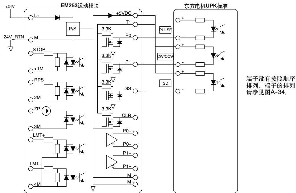
图A-38 连接EM253位控模块和一个东方电机UPK标准
