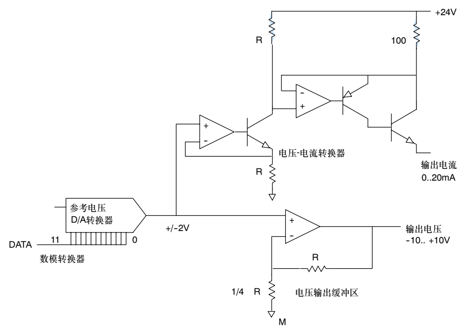
图A-21 EM232和EM235的输出方框图
