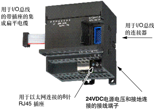
图A-41 连接（CP 243-1 IT）因特网模块
