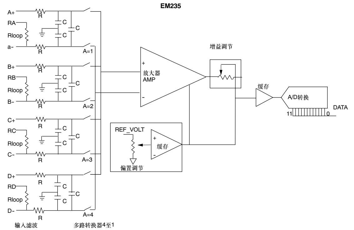
图A-19 EM235的输入方框图
