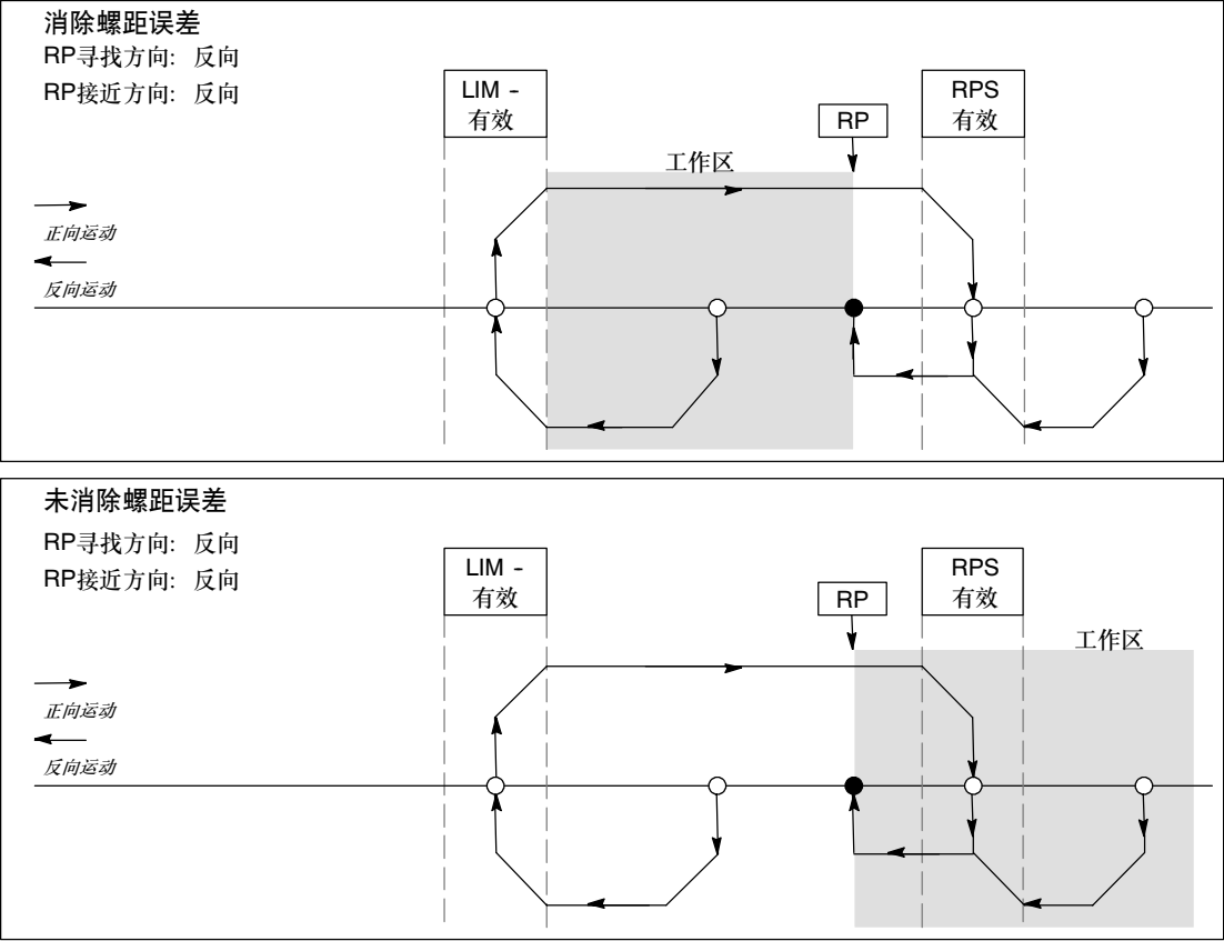
图9-25 消除螺距误差和未消除螺距误差的工作区位置
