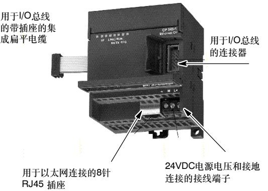
图A-40 连接（CP 243-1）以太网模块
