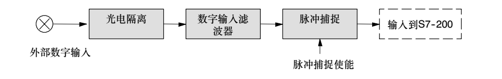
图4-26 数字量输入电路
