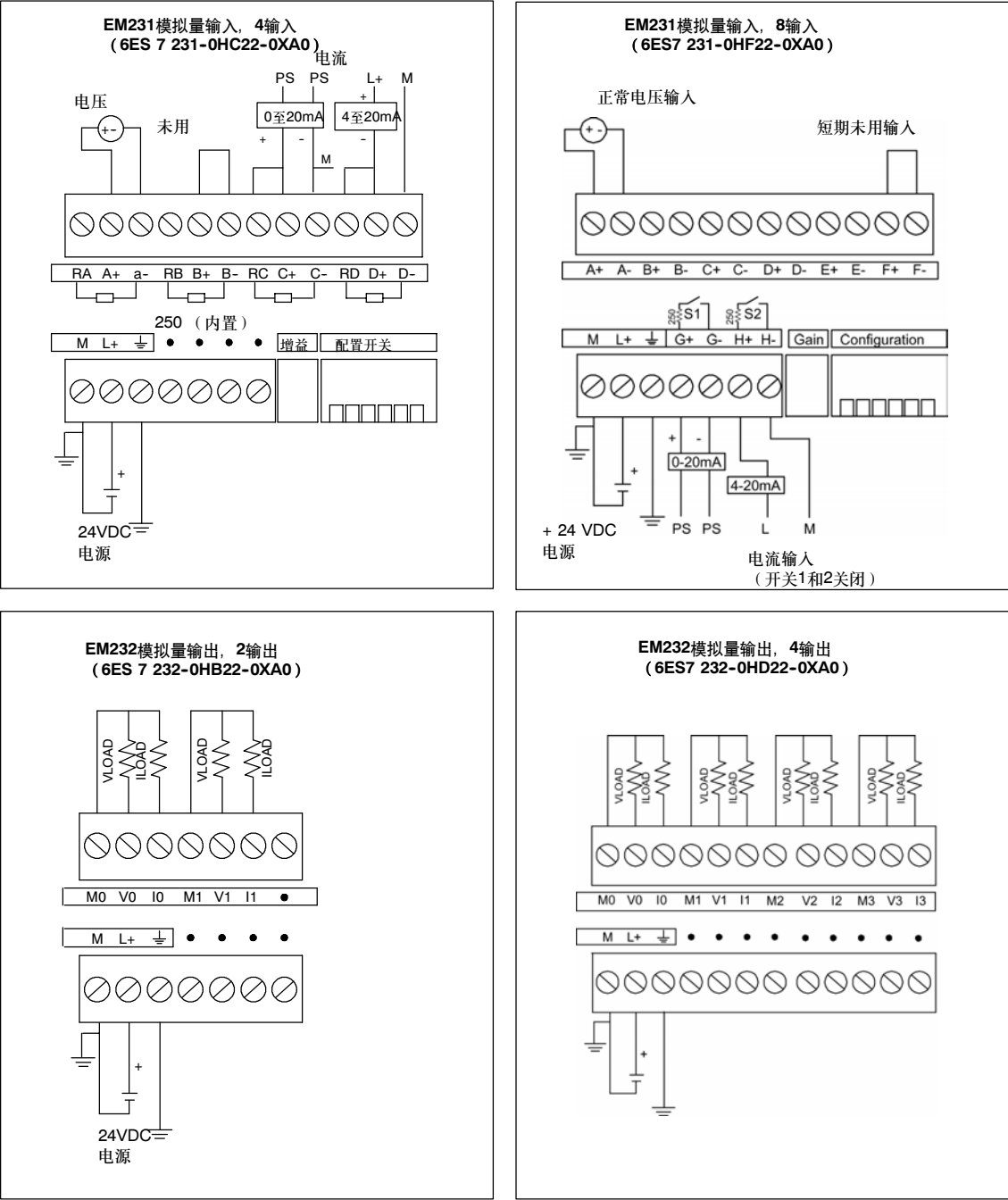
图A-13 模拟量扩展模块的接线图
