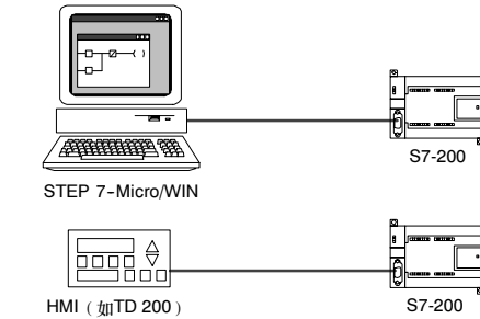
图7-10 单主站PPI网络
