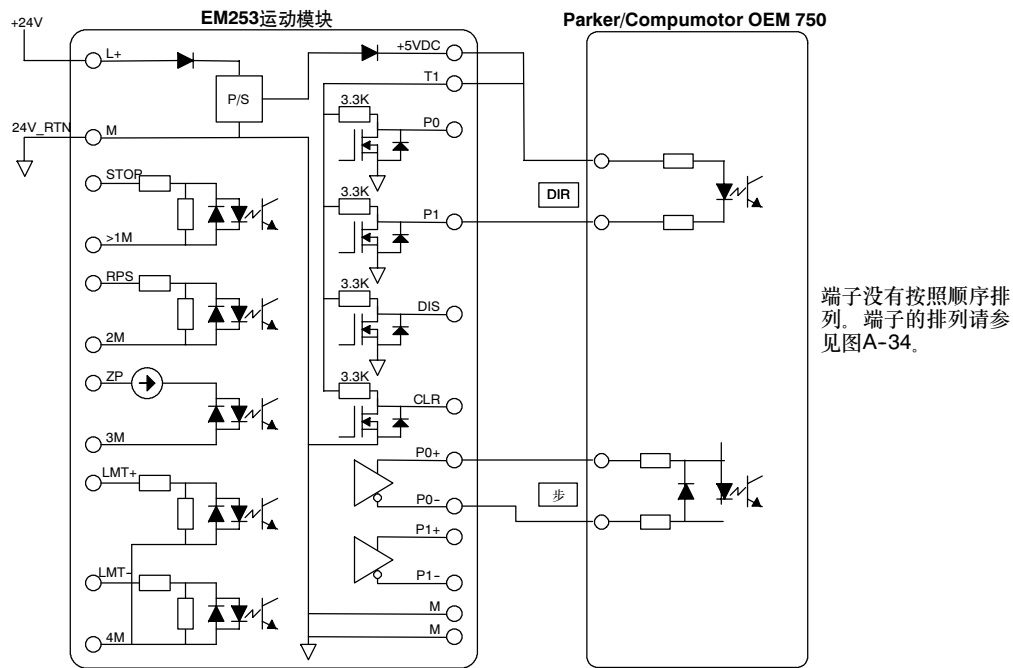
图A-39 连接EM253位控模块和Parker/Compumotor OEM 750
