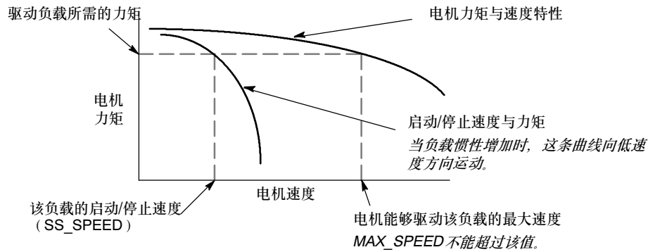
图9-4 典型电机力矩-速度曲线
