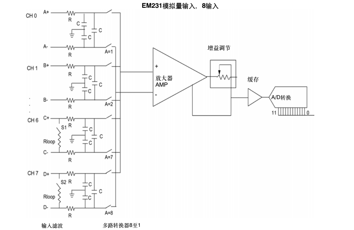
图A-18 EM231模拟量输入的输入方框图，8输入
