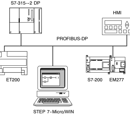
图7-18 PROFIBUS网络
