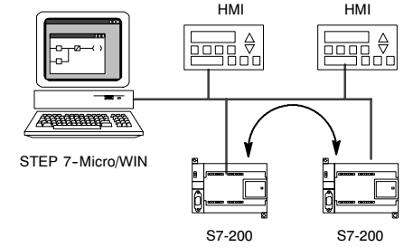
图7-14 HMI设备及点到点通讯
