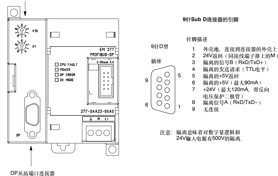
图A-26 EM277 PROFIBUS-DP
