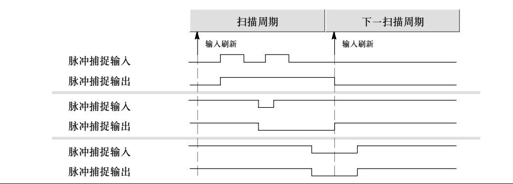
图4-27 不同输入条件下的脉冲捕捉响应
