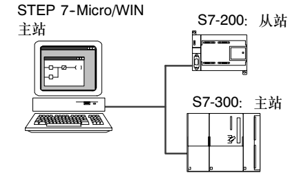
图7-8 MPI网络
