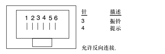
图A-33 RJ11插座的视图
