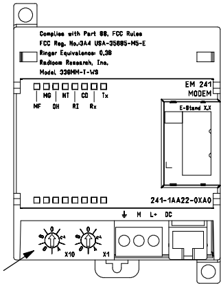
图A-32 EM241 Modem模块接线端子图
