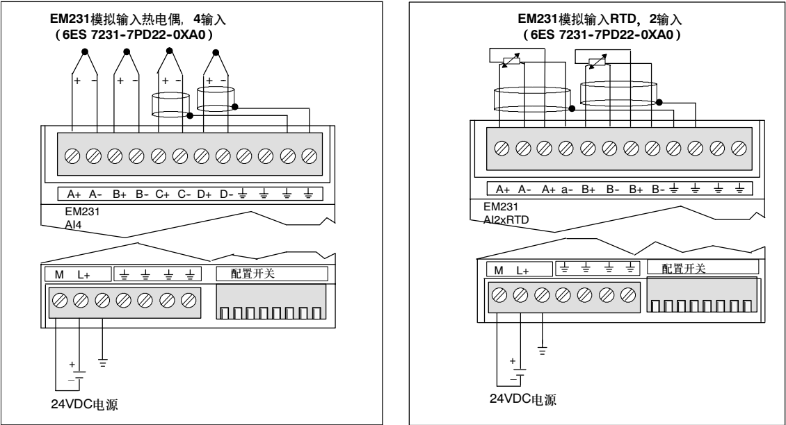
图A-23 EM 231热电偶和EM 231RTD模块的接线端子标识
