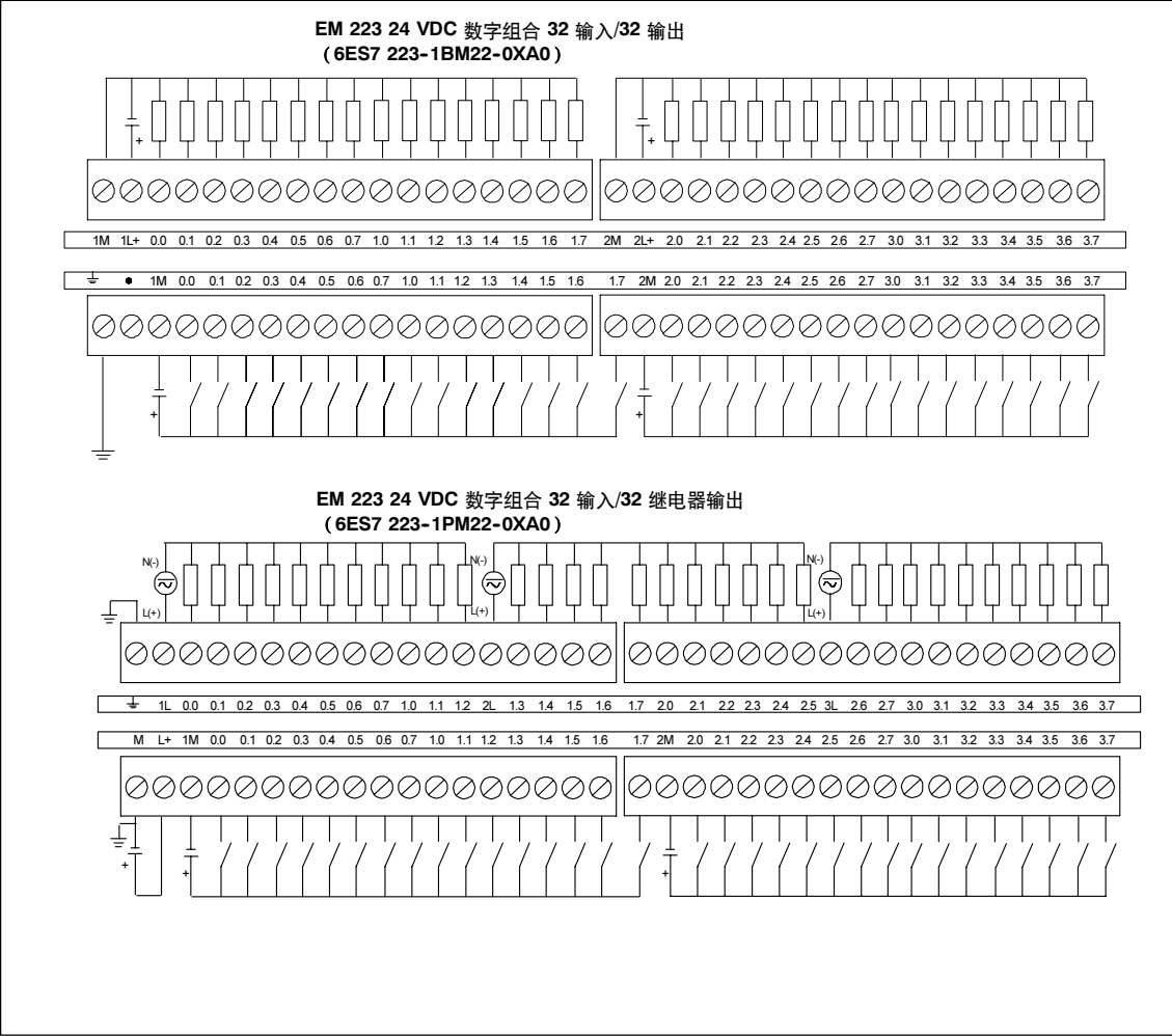
图A-12 EM 223 扩展模块的接线图
