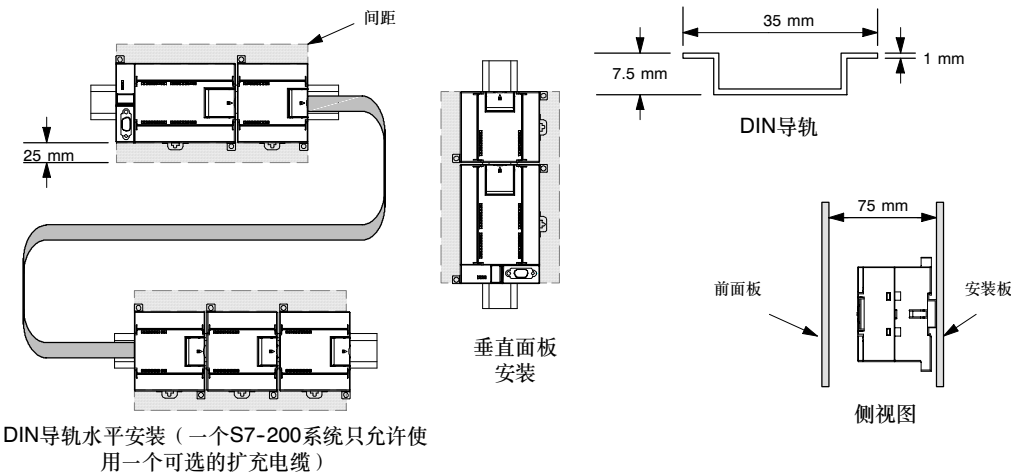
图3-1 安装方式、方向和间距
