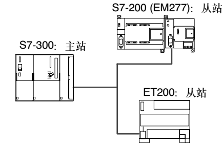
图7-9 PROFIBUS网络
