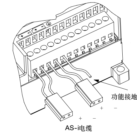
图A-42 CP243-2通讯处理器接线
