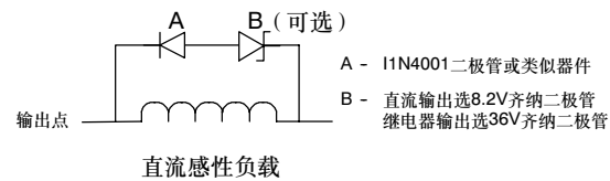
图3-3 直流负载的抑制电路
