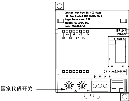
图10-1 EM241调制解调模块
