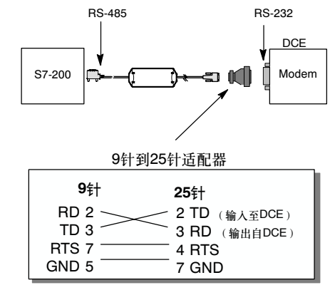
图7-30 适配器引脚分配
