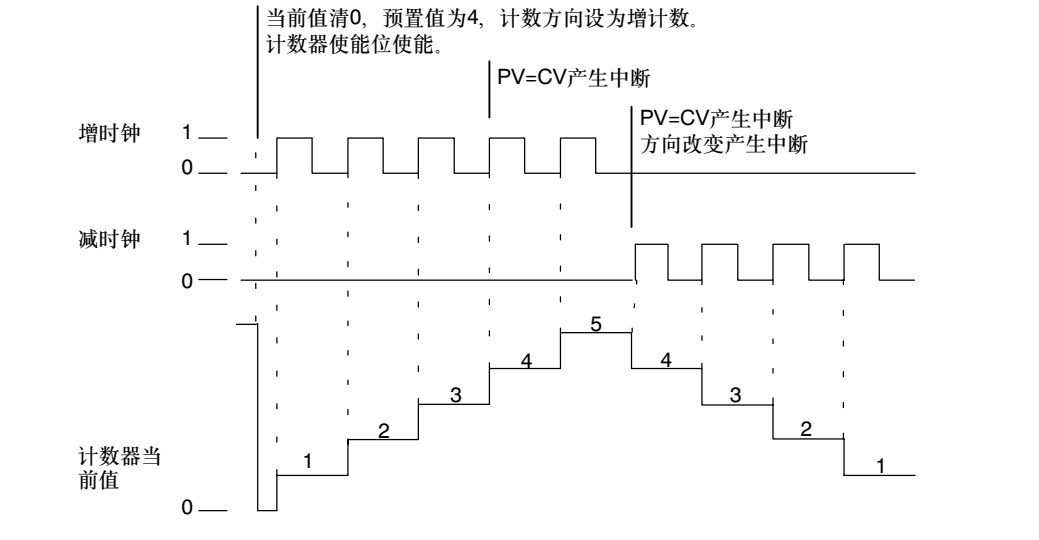
图6-24 模式6、7或8操作实例
