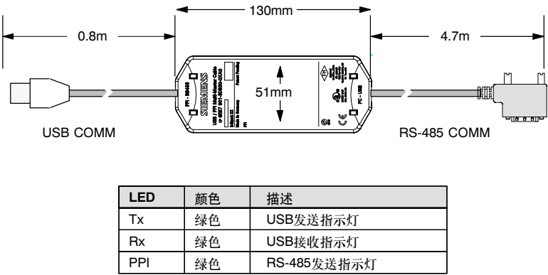
图A-45 S7-200 USB/PPI多主站电缆的尺寸和LED
