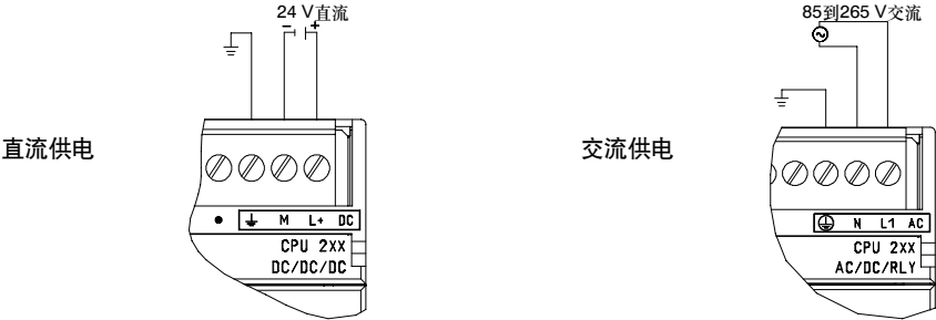
图2-1 给S7-200 CPU供电
