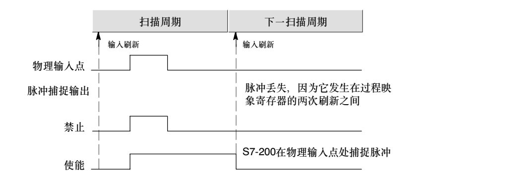
图4-25 带有和不带有脉冲捕捉功能的S7-200操作
