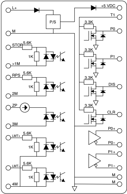
图A-35 EM253位控模块输入和输出内部示意图
