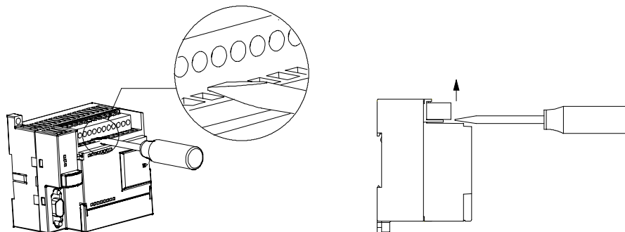
图3-2 拆卸端子排
