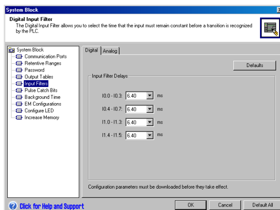
图4-22 数字输入滤波器
