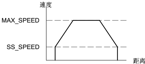
图9-3 最大速度和启动/停止速度
