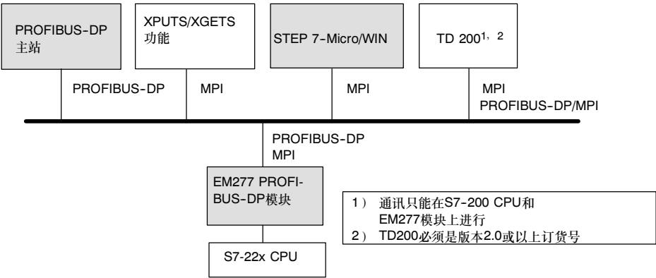
图A-30 PROFIBUS-DP/MPI网络
