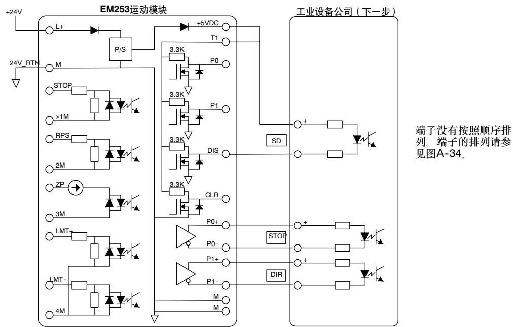
图A-37 连接EM253位控模块到工业设备。（下一步）
