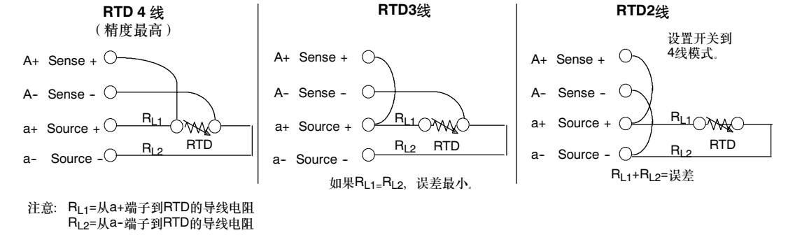
图A-25 RTD到传感器的接线，4线、3线和2线
