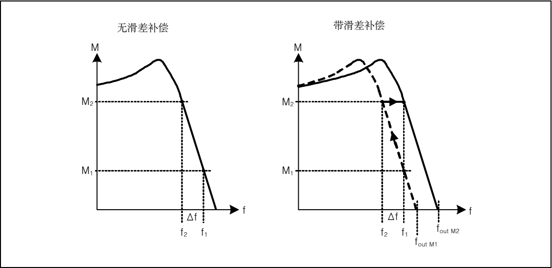
图 3-75 滑差补偿
